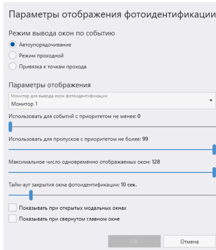
Рис. 11. Общие параметры отображения фотоидентификации
