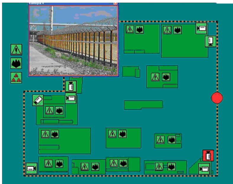
Рис. 16. Отображение различных графических элементов на плане
