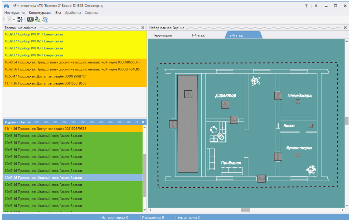
Рис. 6. Режим настройки интерфейса модуля «Бастион-3 – Пост охраны»
