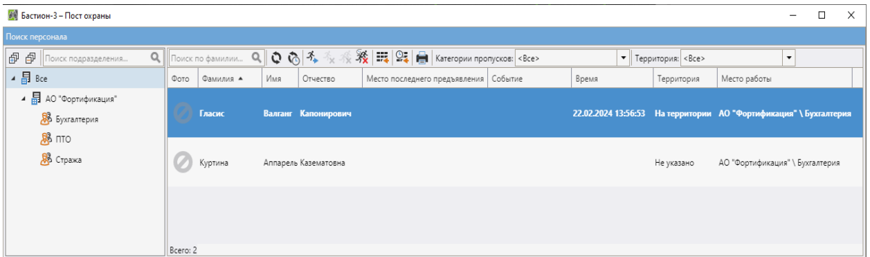
Рис. 37. Окно поиска персонала
