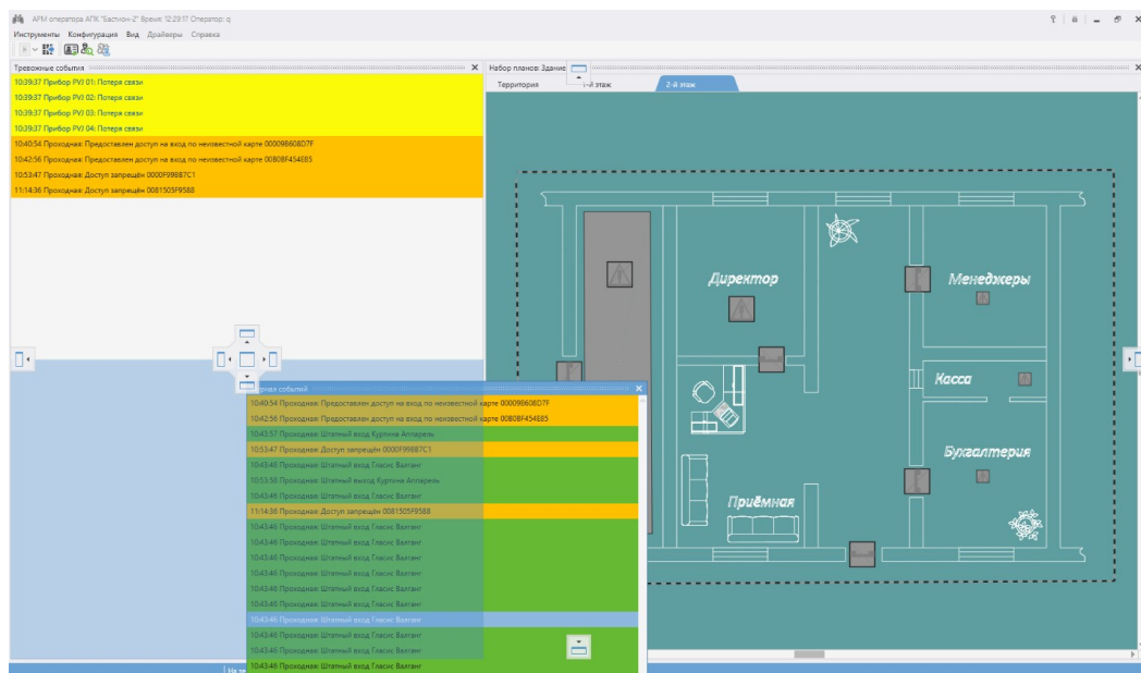
Рис. 7. Режим докинга
