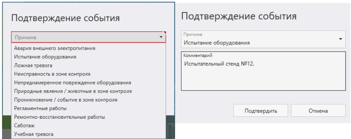
Рис. 14. Запрос причины возникновения события при подтверждении
