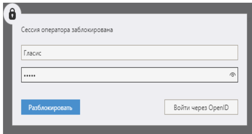
Рис. 4. Окно блокировки
